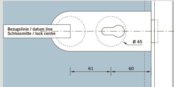
Ansicht Schloss Studio Rondo view lock Studio Rondo
