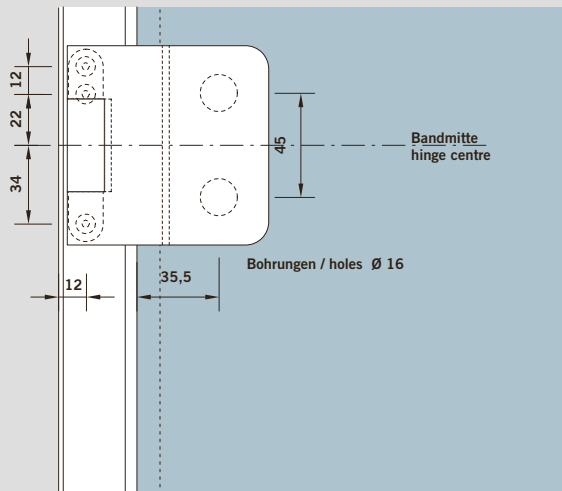
Studio Rondo mit Anschraub-Rahmenteil Studio Rondo with screw-on frame pivot
