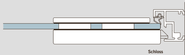
Ansicht Schloss Studio Rondo view lock Studio Rondo
