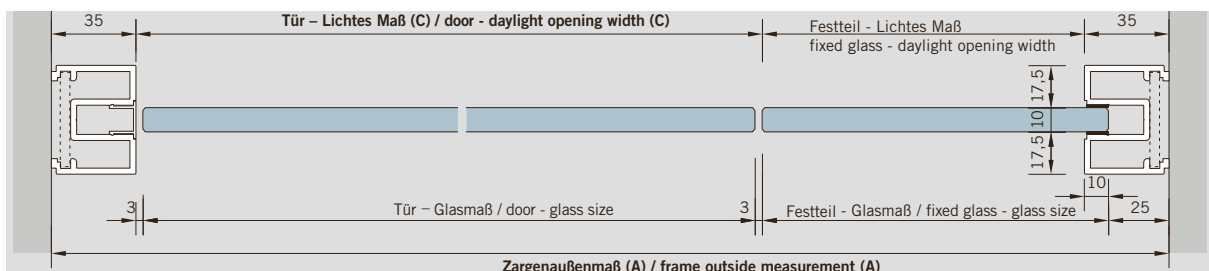
Grundriss / Tür mit Festverglasung / plan / door with fixed glazing
