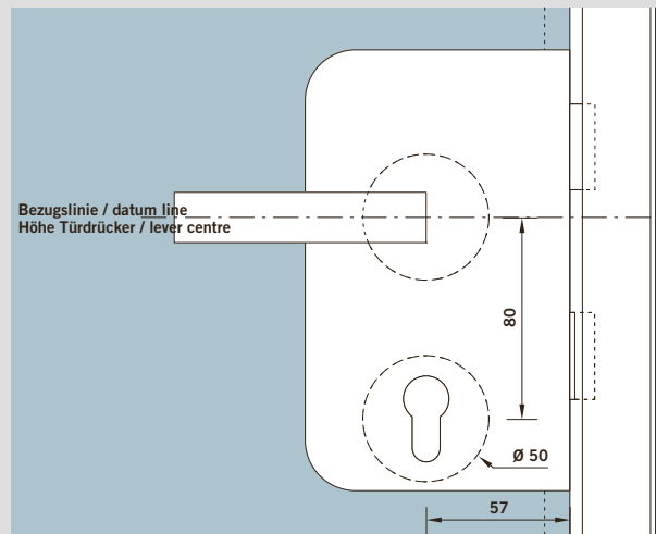
Ansicht Schloss Junior Office view lock Junior Office
