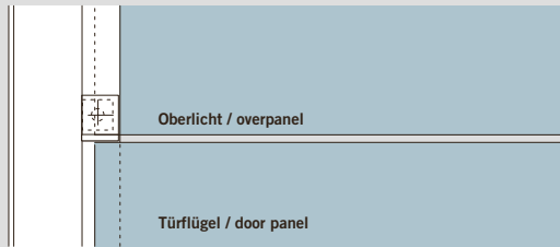
Oberlichtbefestigung / overpanel fixing Haltewinkel justierbar / adjustable angle bracket
