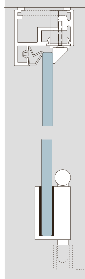
Zargenprofil Frame profile
