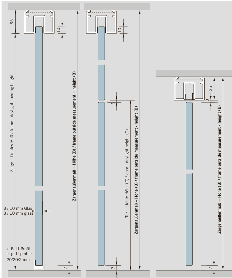
Schnitt / Festverglasung sectional cut / fixed glazing
