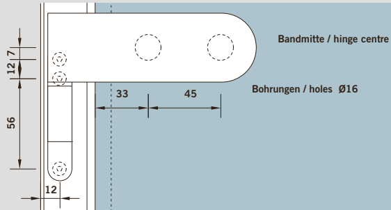
Oberlichtbefestigung / overpanel fixing Haltewinkel justierbar / adjustable angle bracket
